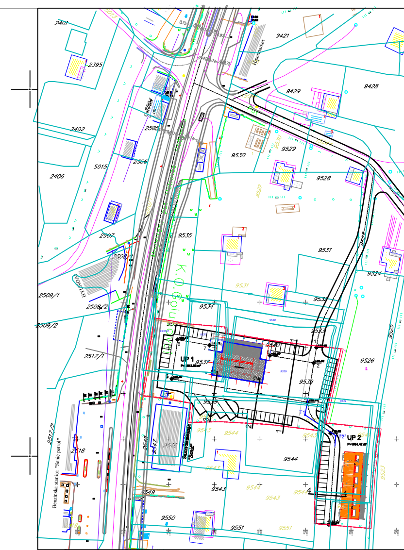
VEZA PREDMETNE LOKACIJE SA ŠIROM SAOBRAĆAJNOM MREŽOM R 1:2500
