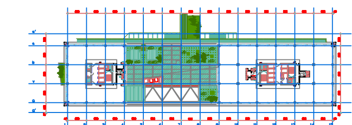
c) osnova karakteristične etaže
