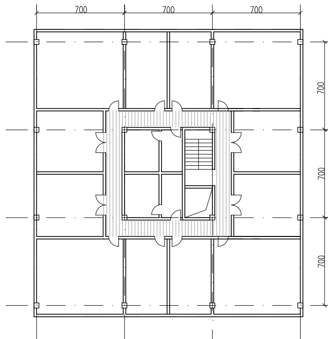
Osnova prvog i drugog sprata
