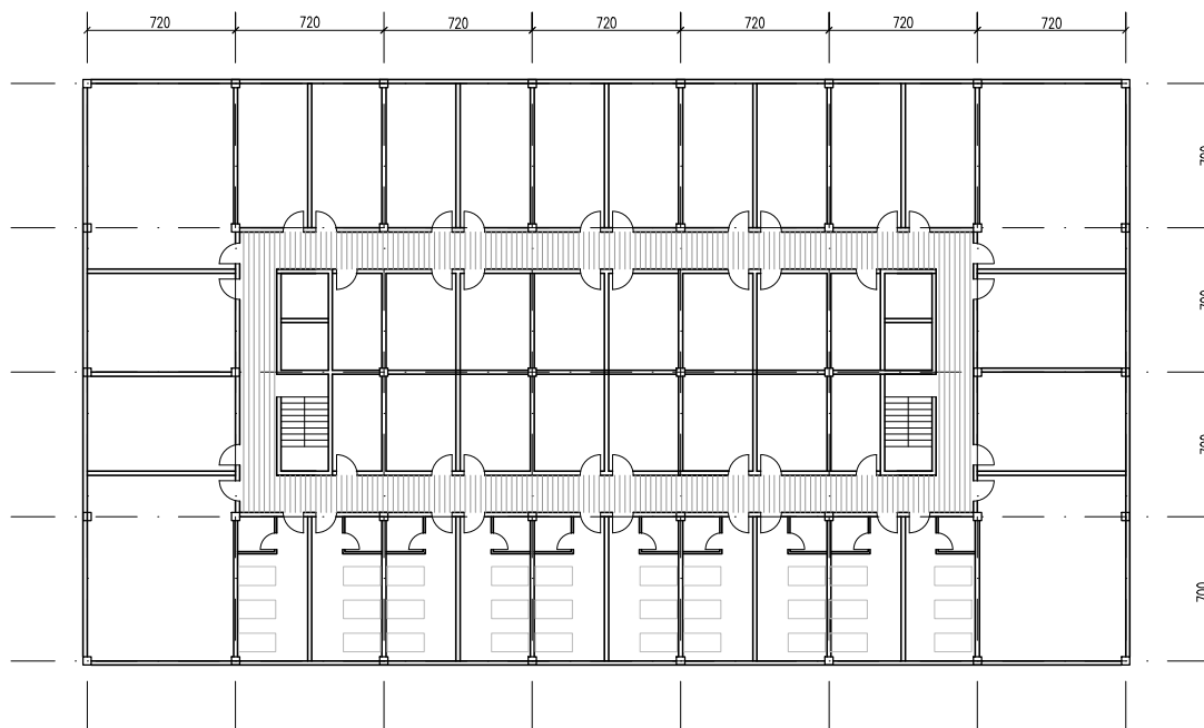
Osnova prvog i drugog sprata
