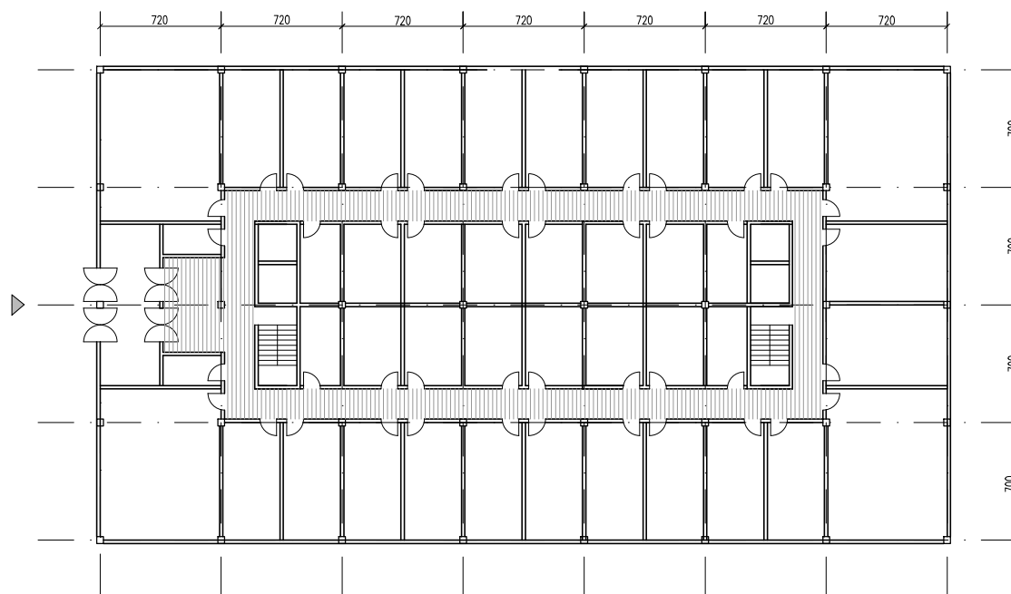
Osnova prizemlja
