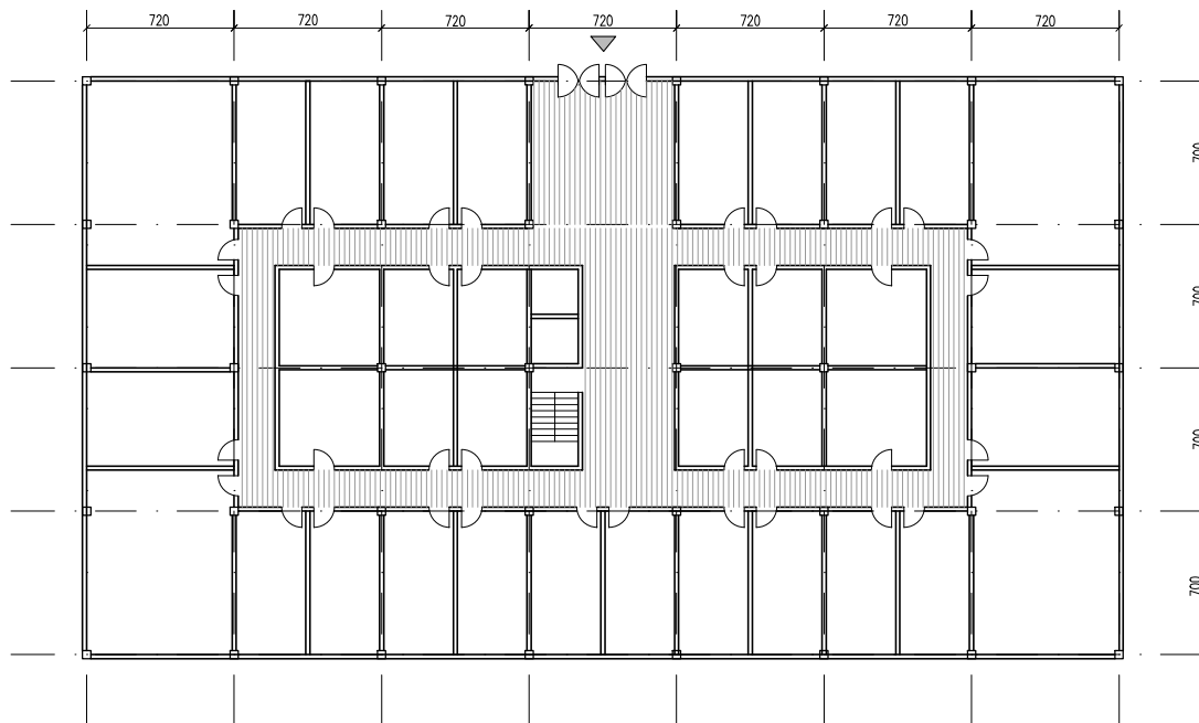
Osnova prizemlja
