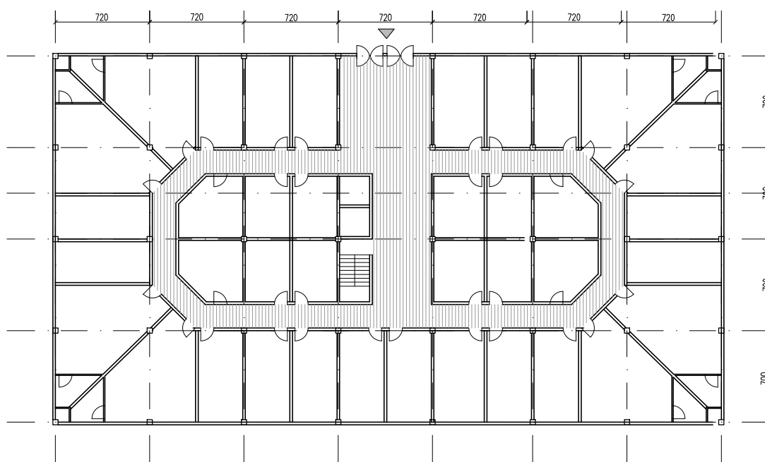
Osnova prizemlja
