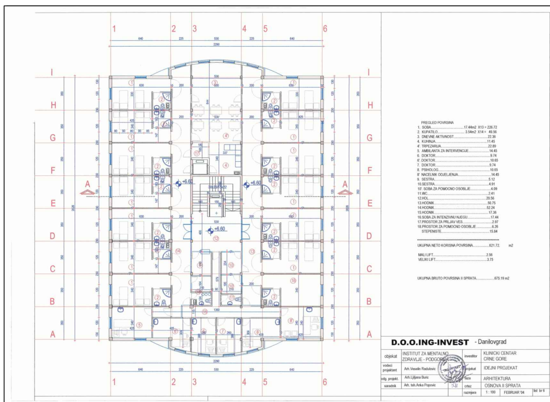
Osnova drugog sprata
