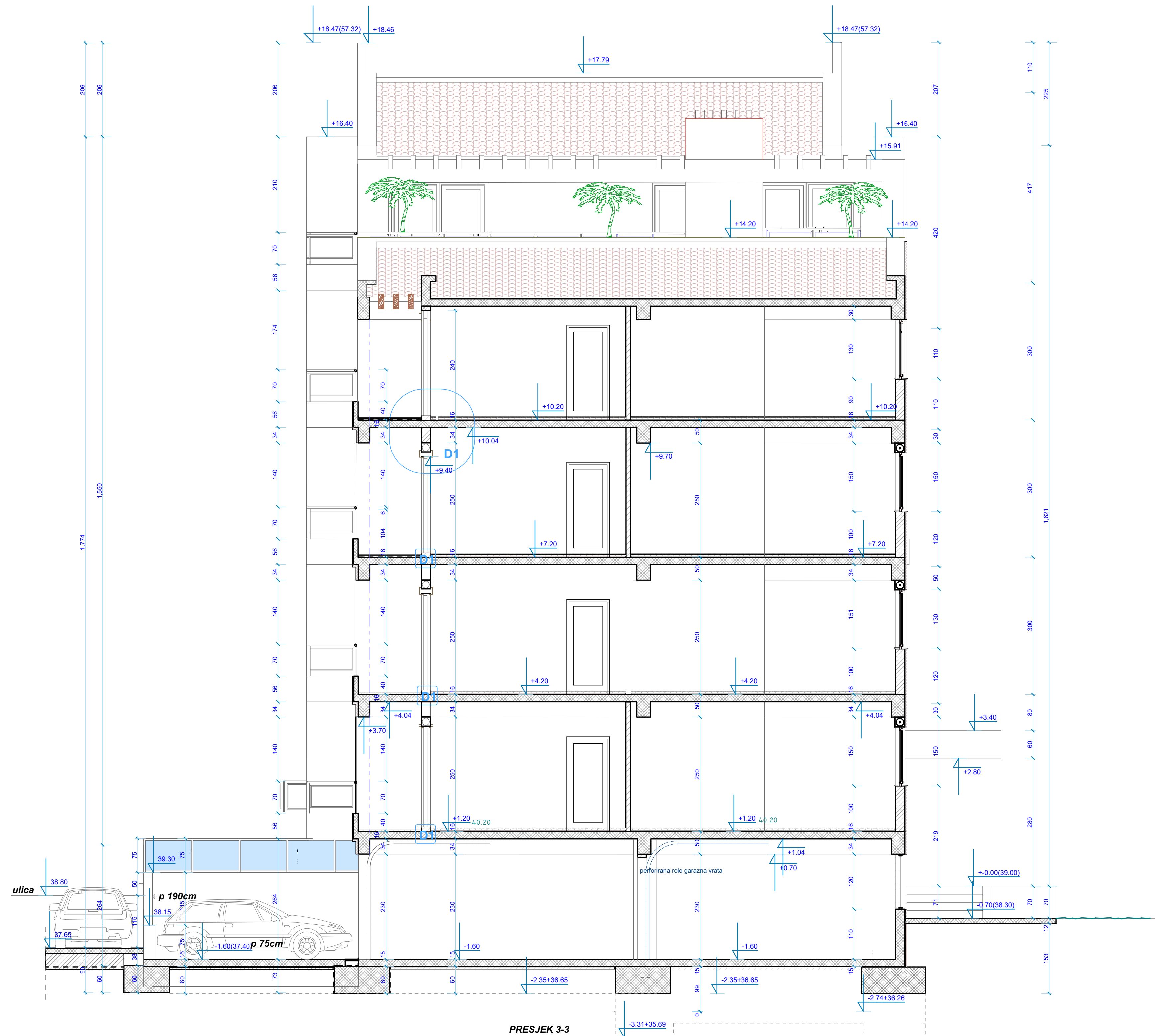
PRESJEK 3-3
