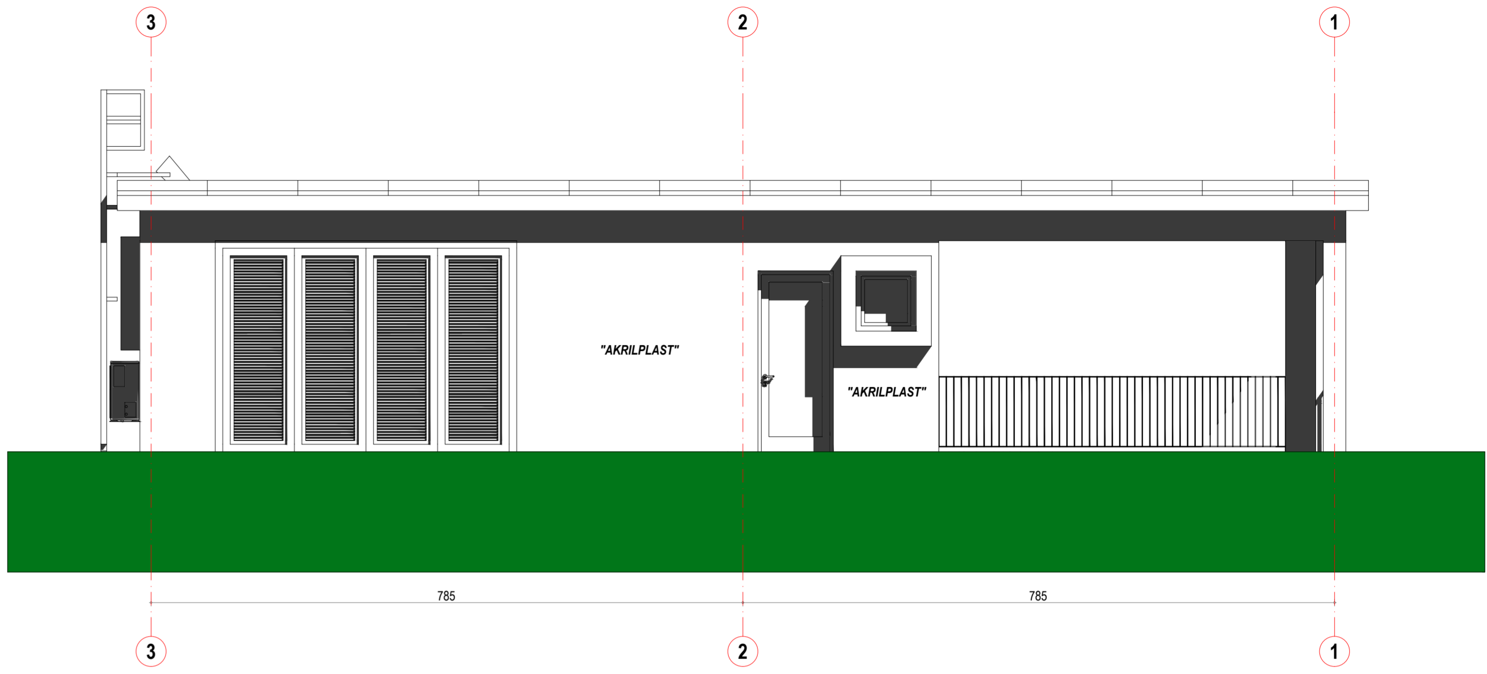
SJEVERNA FASADA
